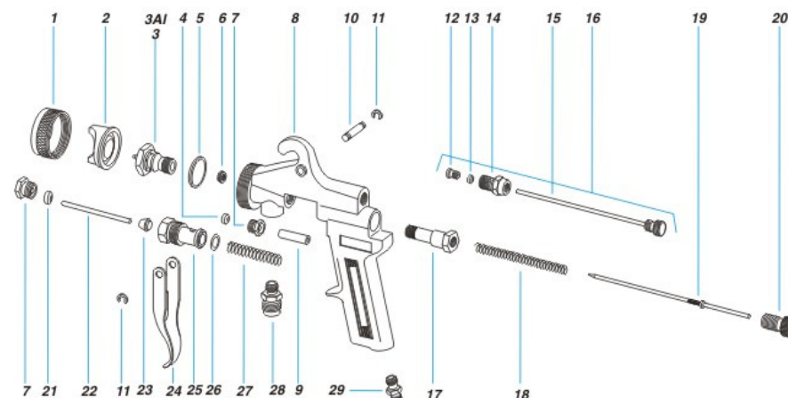
MODELO 1A/1AI TAMPA EM ALUMÍNIO
